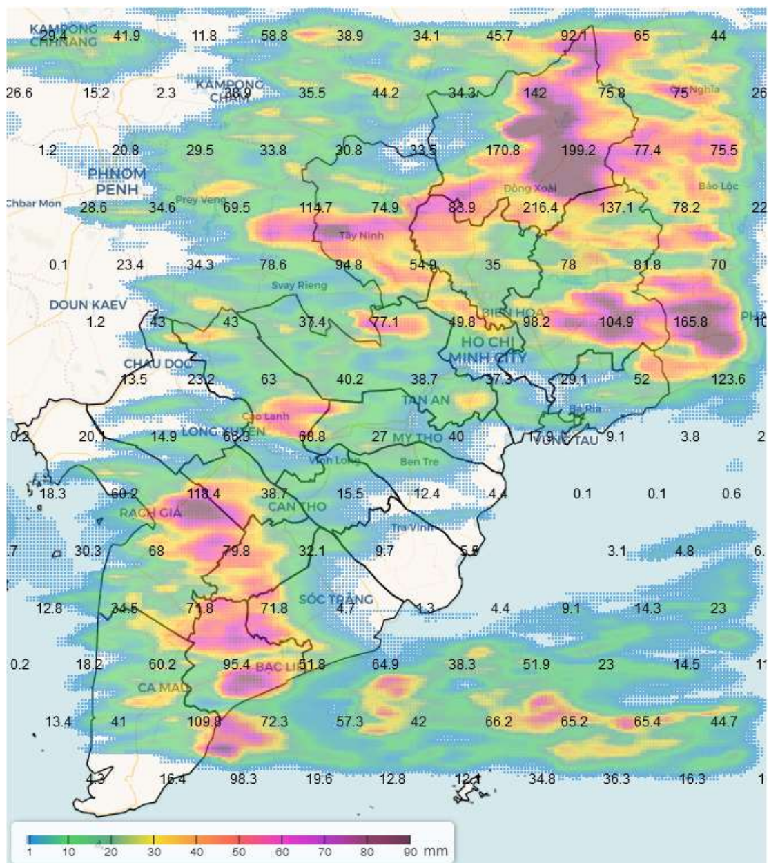
Bản đồ dự báo mưa từ 19h ngày 08/6 ngày 19h ngày 09/6 ở khu vực Nam Bộ
